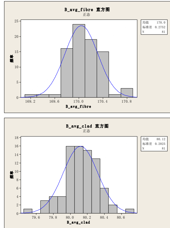
图 3 长飞公司 BI1015-B 系列光纤涂覆层和包层统计数据
