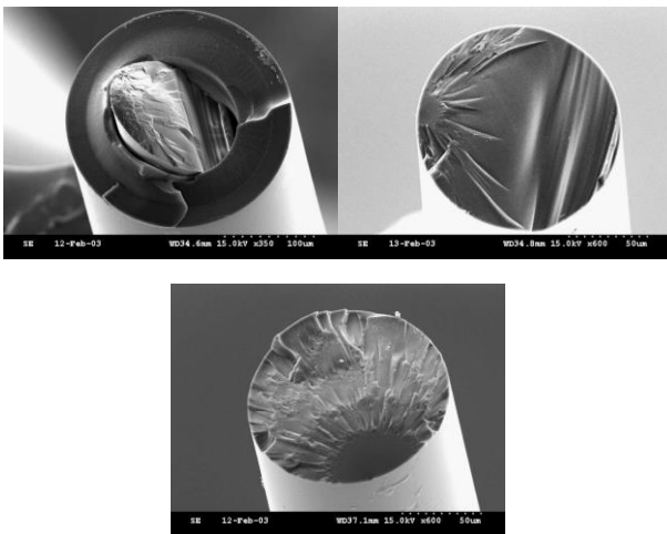
图 2 光纤在不同应力下的断裂端面图（应力从左到右变小）
