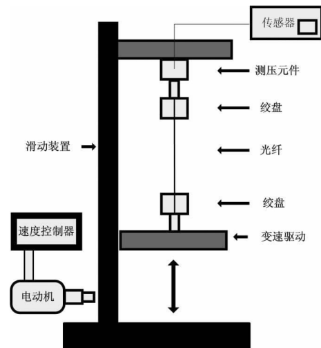
图 1 位移式测试装置
