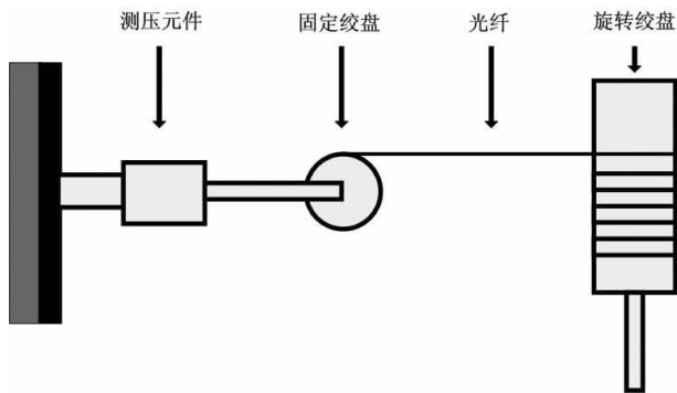
图 2 旋转式测试装置
