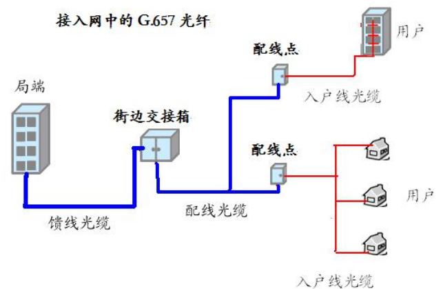
图 1 G. 657. A1 和 G. 657. A2 类光纤在接入网中的应用
