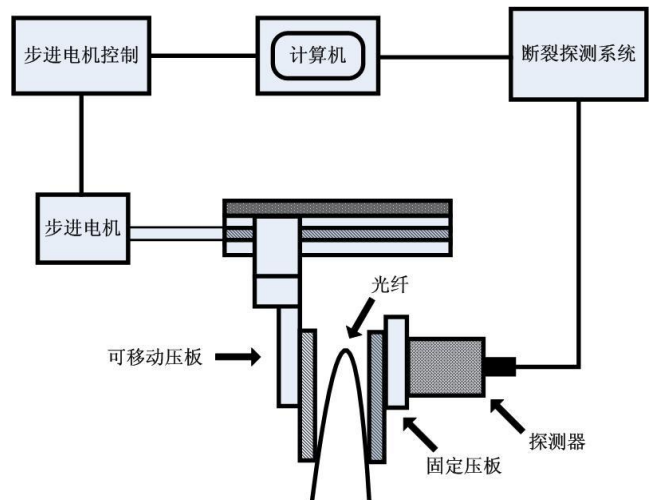
图 1 两点弯曲装置示意图
